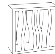
Poisson
