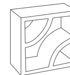
Tramontane
