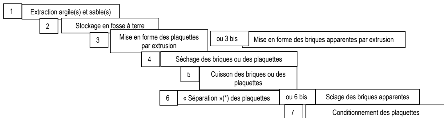
Sch ma d crivant le proc d  classique de fabrication des plaquettes
